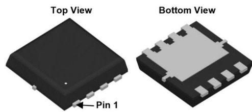
PDFN3x3-8L
